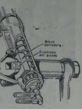
Fig. 4. Una nueva dirección Americana "Hannum" en la cual el esfuerzo de palanca es variable, siendo el mínimo en la posición del centro. Esto es efectuado por una leva desplazable.
