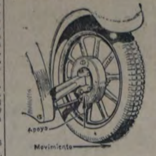
Fig. 5. Pivote inclinado que tiende a levantar el coche; la carga produce una acción tendiente a centrar las ruedas automáticamente.
