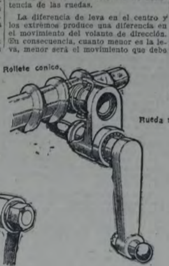
Fig. 6. Un mecanismo a sinfín y rollete de bolas, patentado por Mr. Dixon y la Dalmer Co.
