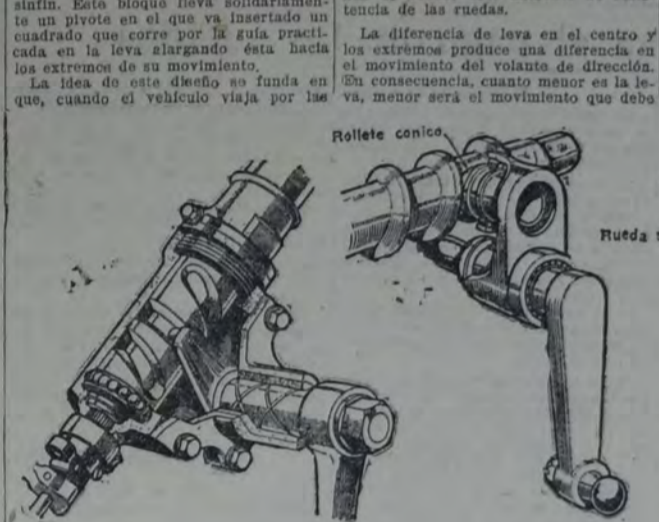
Fig. 5. La dirección Ross, la más empleada en América. La forma especial del sinfín provee una palanca variable.
