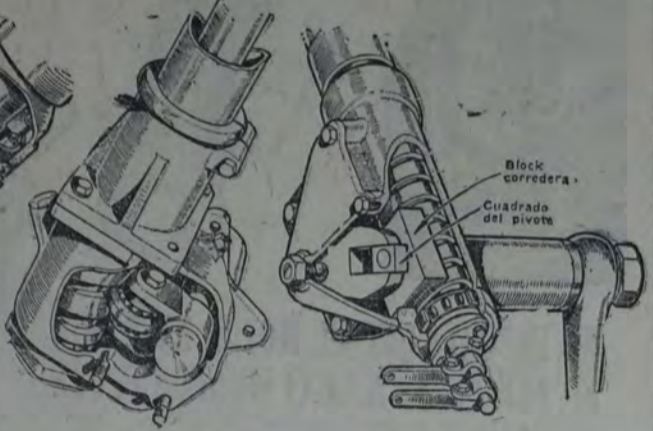
Fig. 3. La bien conocida dirección "Marles", en la cual un rollete engrana con un sinfín especial.
