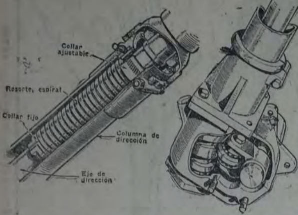
Fig. 2. Un proyecto de resorte en espiral para ayudar a la estabilidad automática de las ruedas, patentado por Mr. F. H. Royce.
