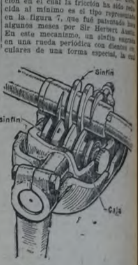
Fig. 7. Un mecanismo ingenioso que usa una rueda periódica sinfín con dientes circulares, patentada por Sir Herbert Austin.
